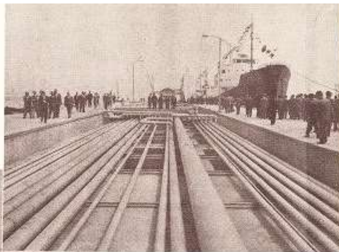
40,000トンのスーパータンカー 2隻が同時荷役の専用大橋
